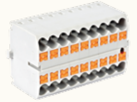
PMIT15 18x2,5
